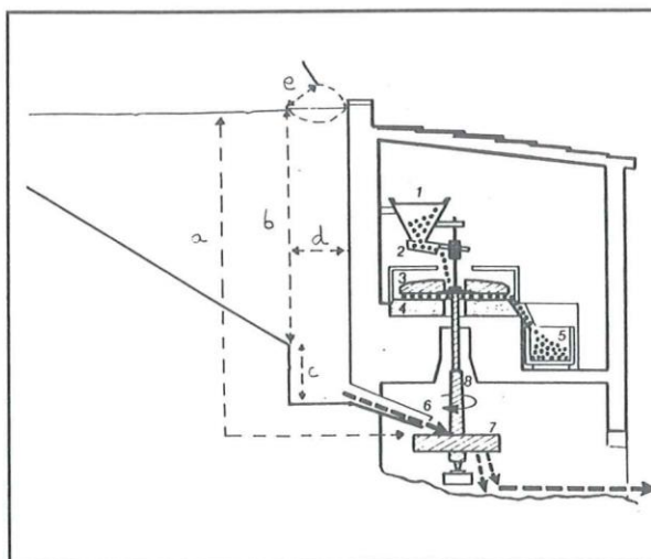
Fig. 4: Esquema d'un molí fariner. El gra, representat per punts grossos, situat a la tremuja (1) cau pel canalot (2) fins a l'ull de la mola, i es fica entremig de la mola volandera (3) i la mola sotana (4). El gra mòlt (farina) surt pel farinal i es recull a la farinera (5).
